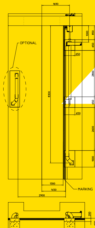
Funderingsafmetingen COMBILOK® SWAP Rechts
